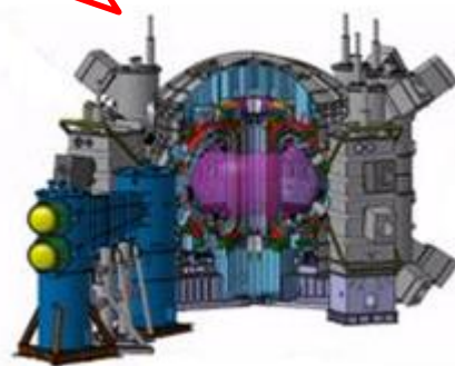
那珂研究所の核融合炉
